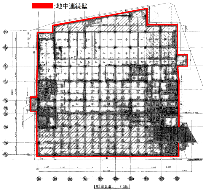
图 3-3 B1 階伏図
