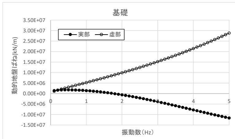
図 4-8 Novak 法による地下側面地盤バネ
