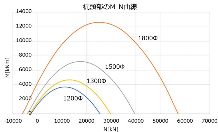
図 5-13 杭頭部の M-N 曲線
