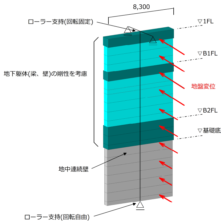
図 3-15 地中連続壁 1 エレメントの解析モデル
