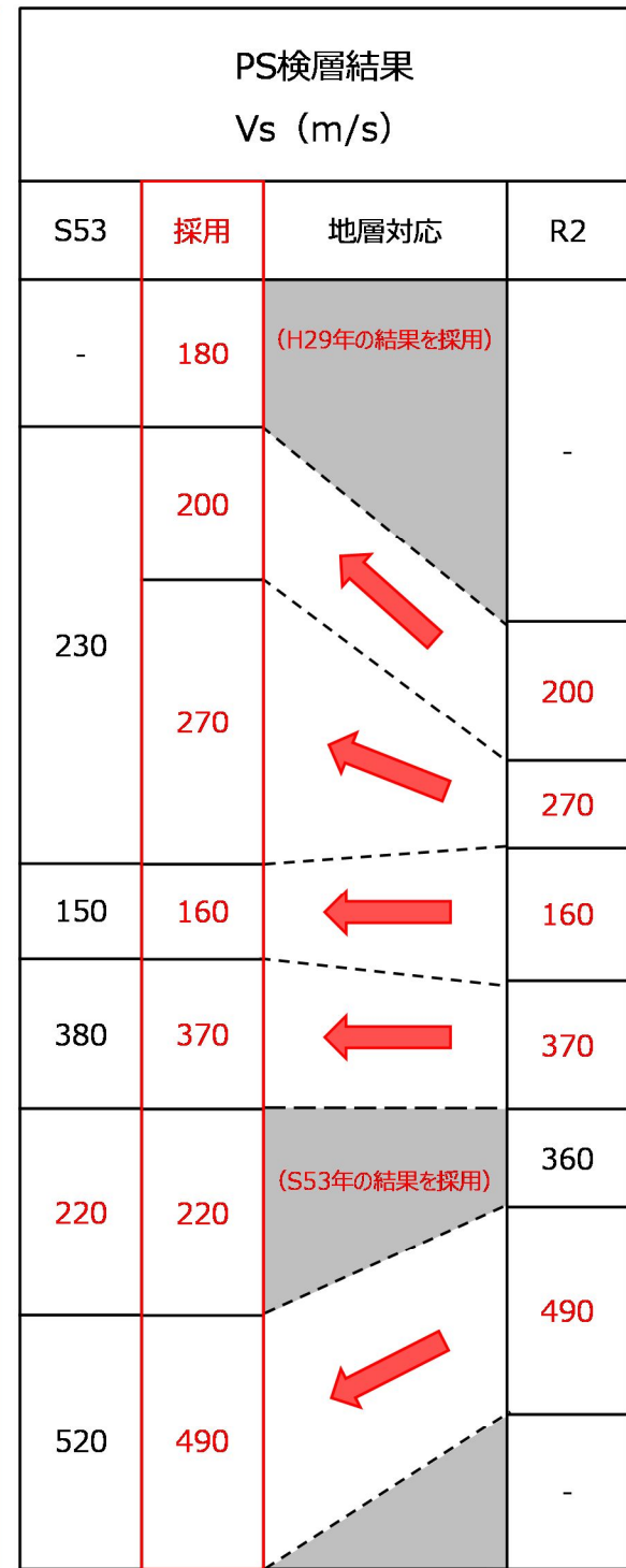
図 2-4 地盤構成と Vs 比較 (左: 昭和 53 年、右: 令和 2 年、赤字: 採用値)
