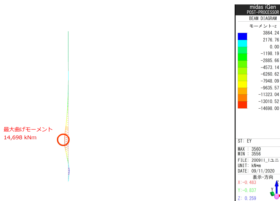
図 3-16 地中連続壁 1 エレメントの検討結果
