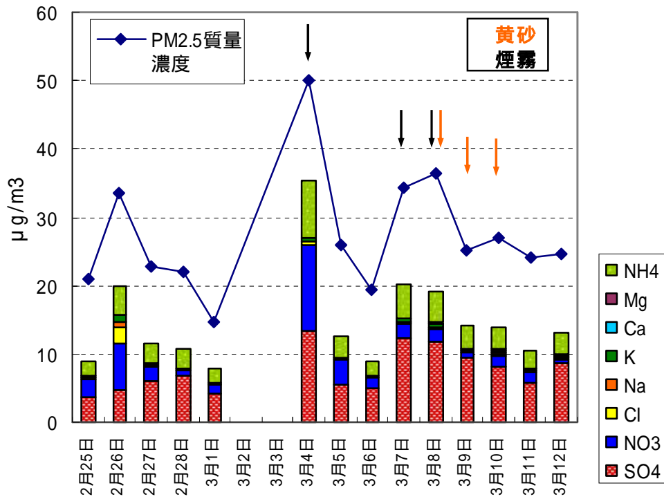
図2 質量濃度とイオン成分濃度の時系列変化
