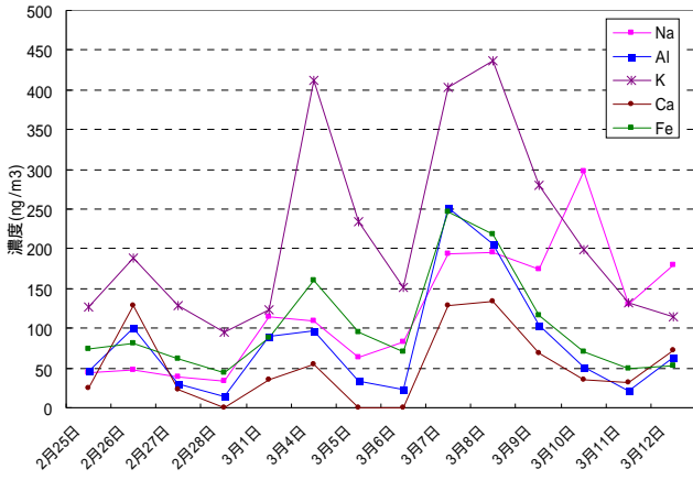
図 6 - 1 各無機元素濃度の時系列変化 1
