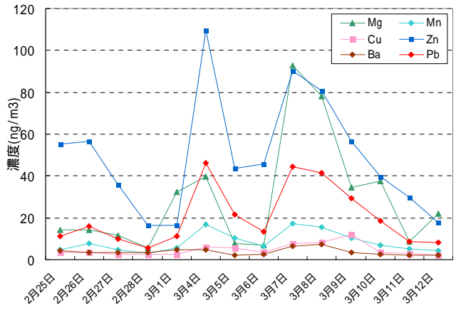
図 6 - 2 各無機元素濃度の時系列変化 2
