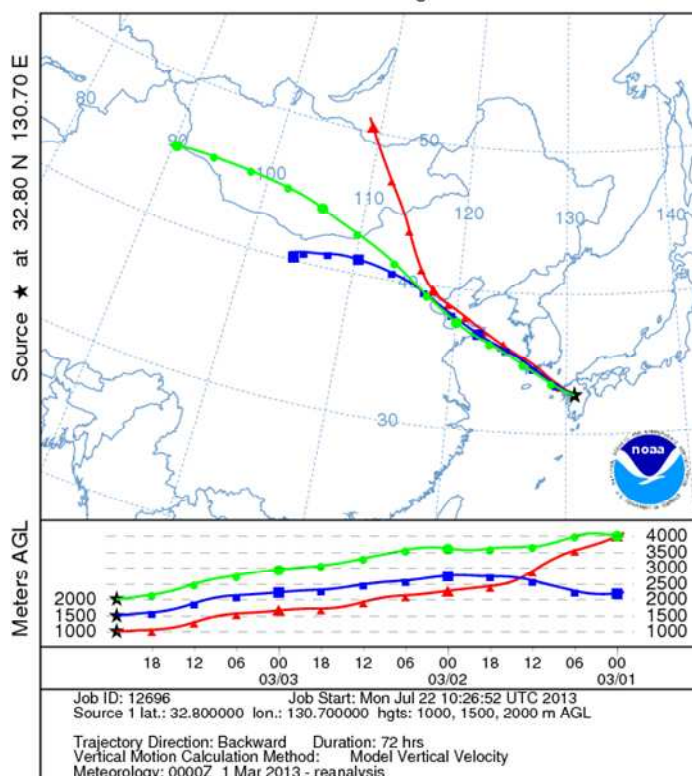
図4 3月4日8時の後方流跡線解析図
