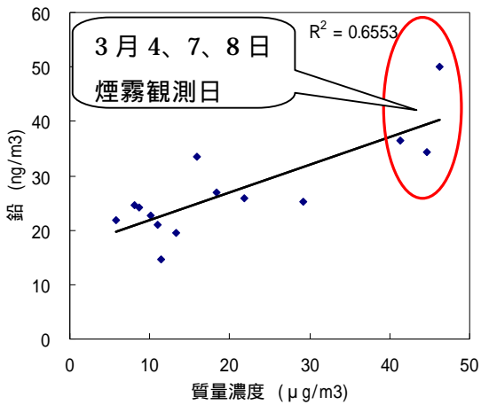
図 8 質量濃度と鉛元素濃度の相関関係
