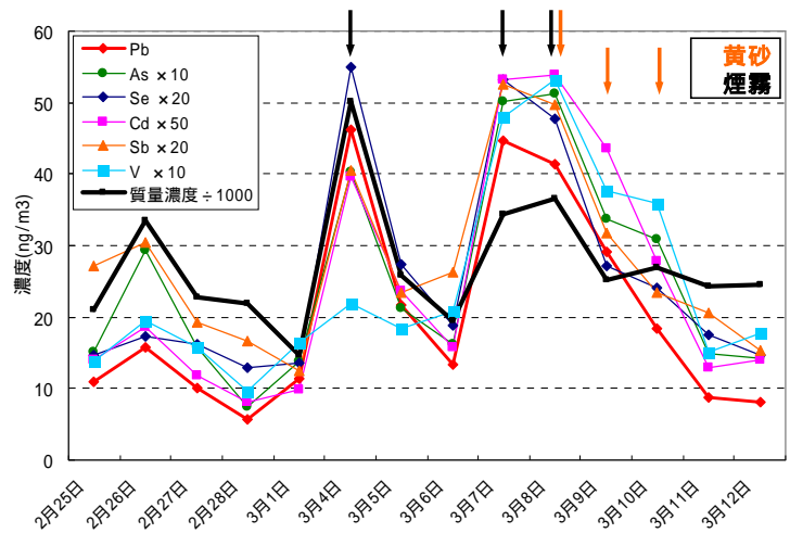
図 7 高濃度日を中心とした各無機元素濃度の割合
