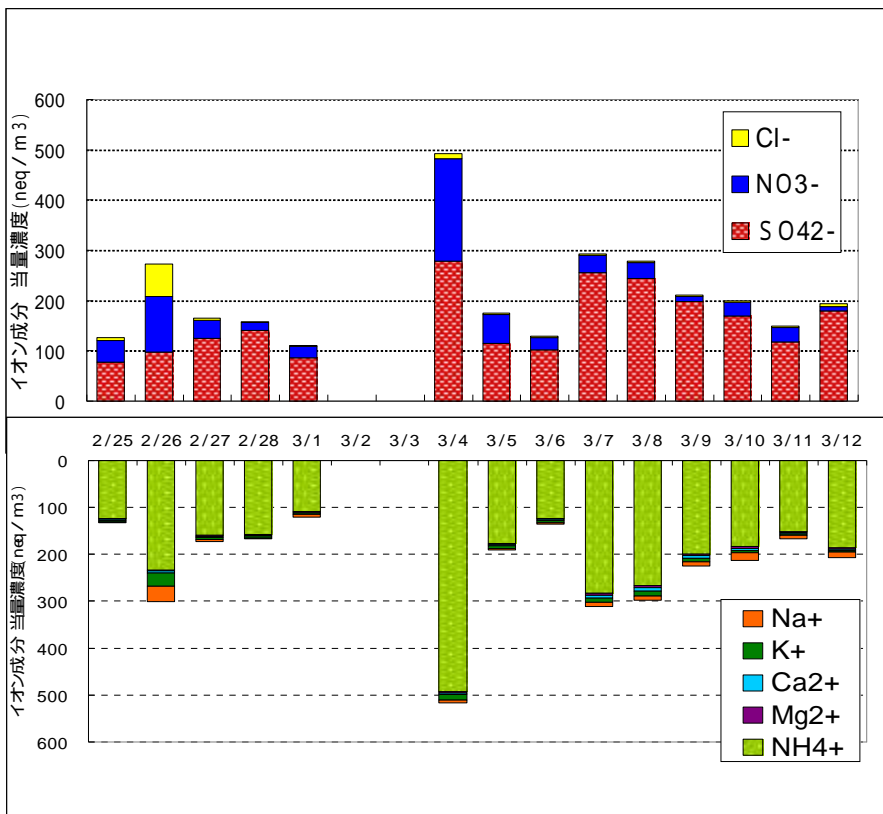
図3 イオン成分の陰イオンと陽イオンの当量濃度比較
