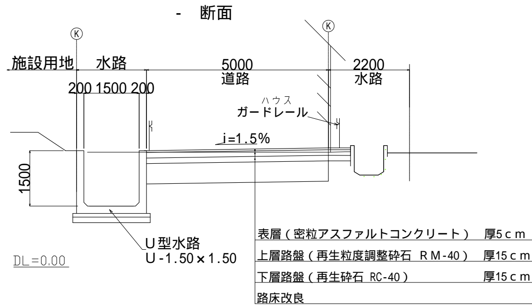
4号水路断面図
