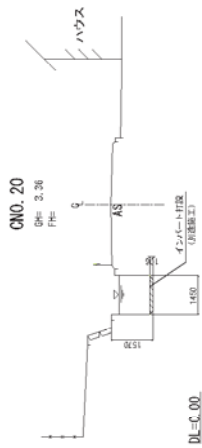
補修断面図
