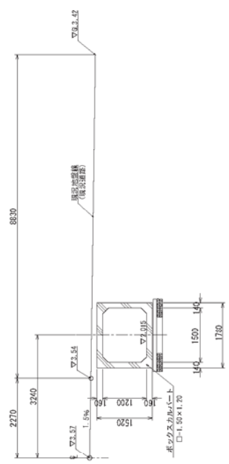
2-2断面図 S=1:50
