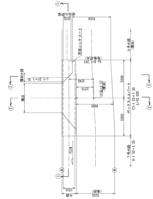
平面図 S=1:100
