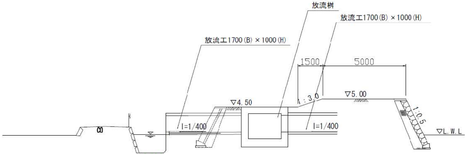
(参考図) 調整池放流部概略断面図
