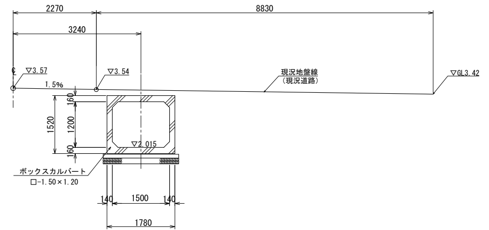
2-2断面図 S=1:50
