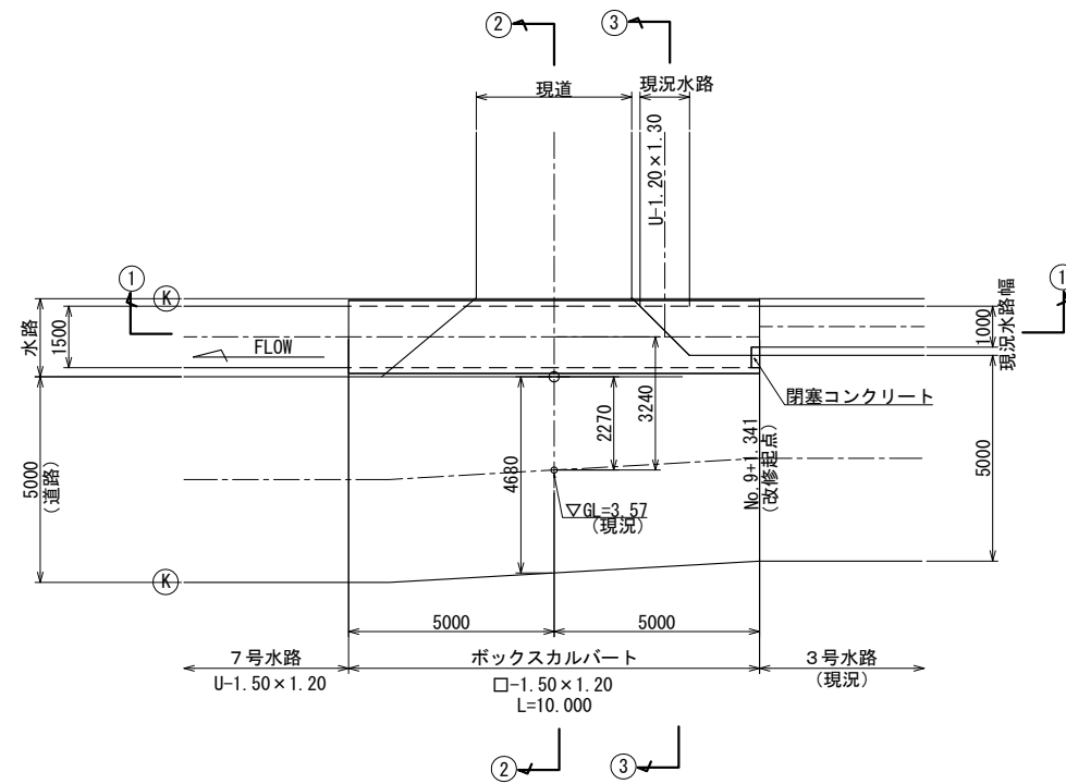
平面図 S=1:100
