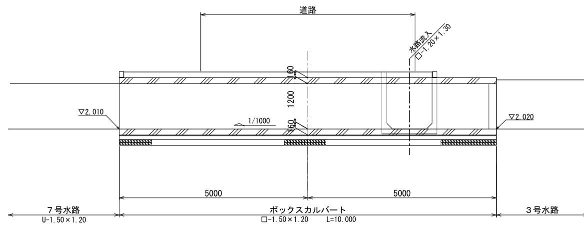
1-1断面図 S=1:50
