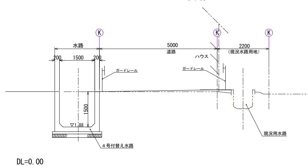
3-3断面図 S=1:50
