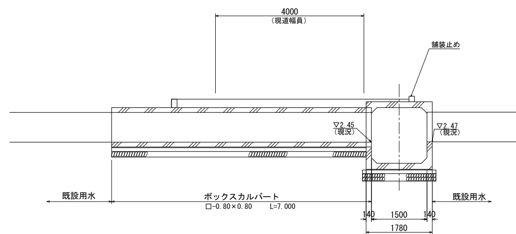
2-2断面図 S=1:50
