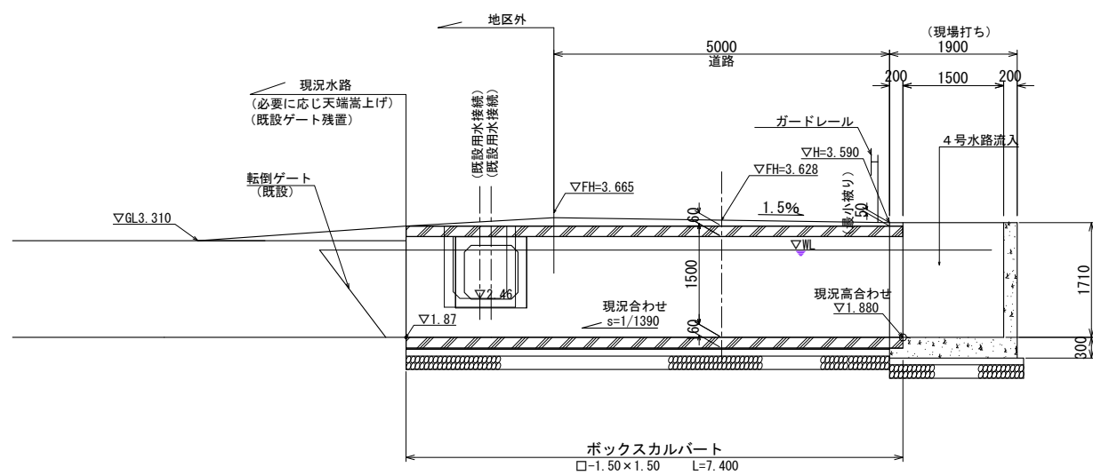
1-1断面図 S=1:50
