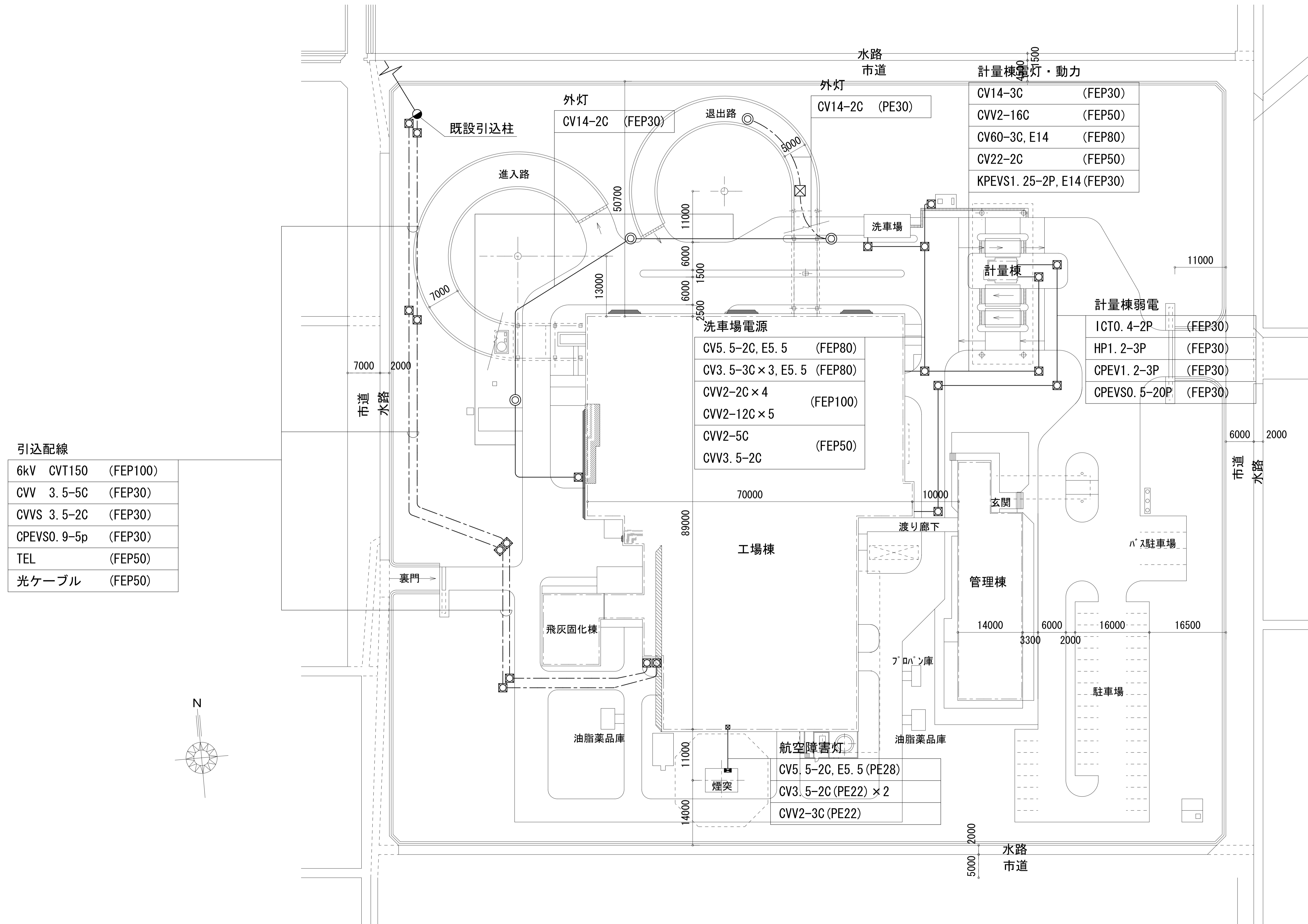
現西部環境工場 屋外配線平面図 S=1/800
