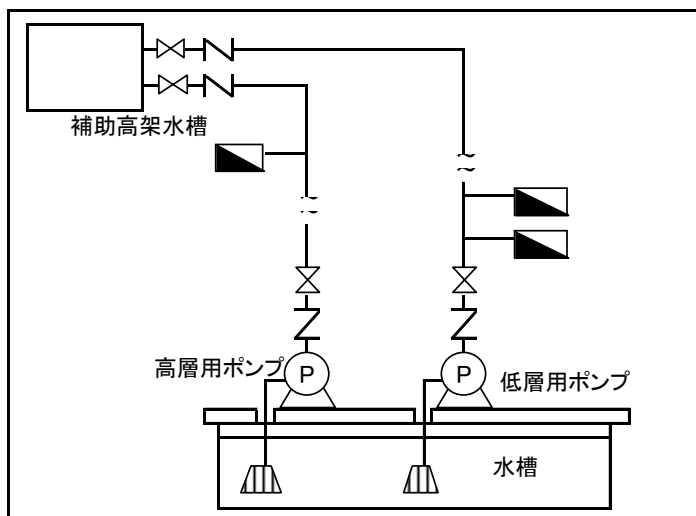
《配管系統を別にした場合の例》
