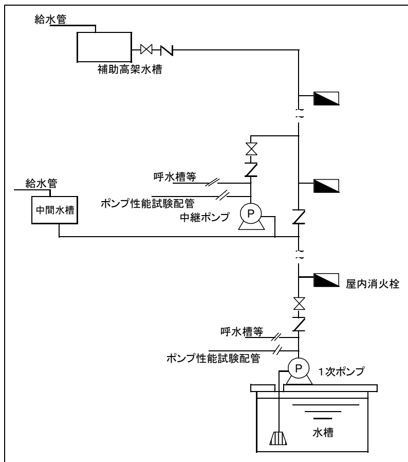
《中継ポンプを設けた場合の例》
