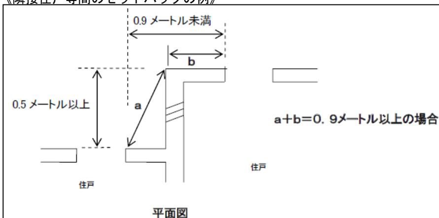
《隣接住戸等間のセットバックの例》
