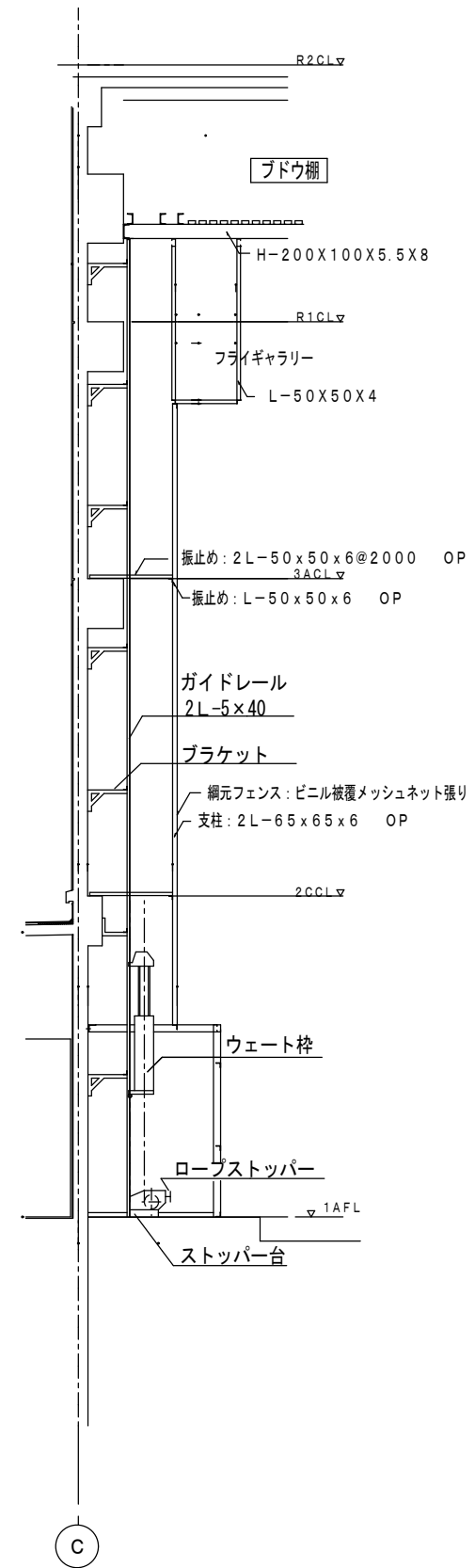
熊本市富合ホール舞台機構設備断面図
