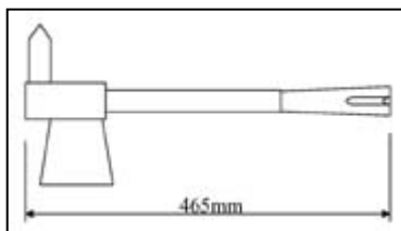
《図3 破壊器具》
