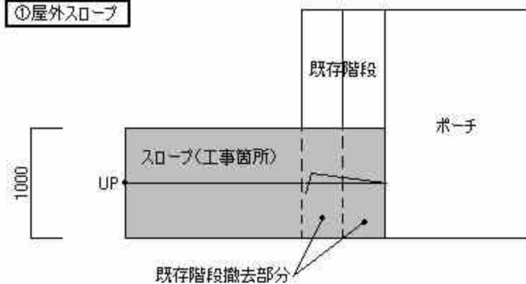
平面図
