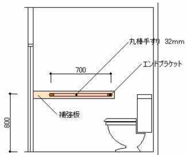
立面図
