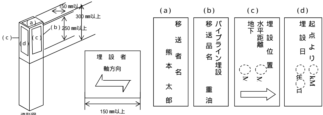
姿形図 (標識柱)
