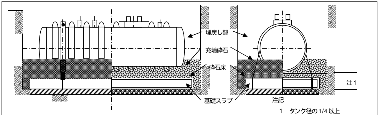
<図1-3 充填砕石施工図>
