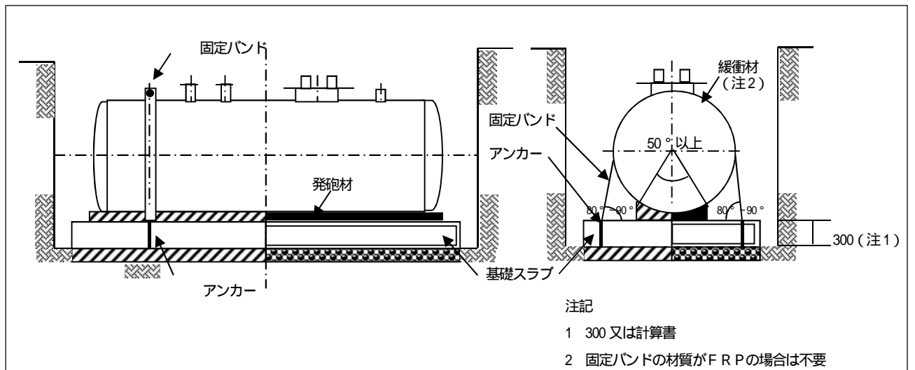
<図 3 - 1 発泡材施工図>
