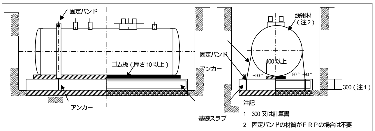
<図2-1 ゴム板施工図>
