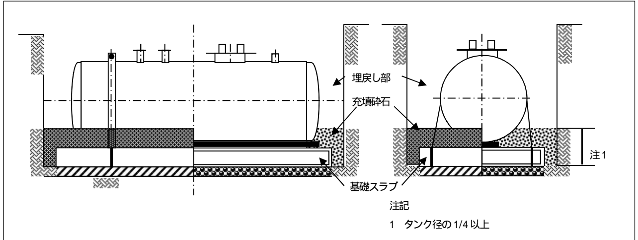
<図 2 - 2 充填碎石施工図> 支持碎石は図 1 - 2 のとおり施工されているものとする。
