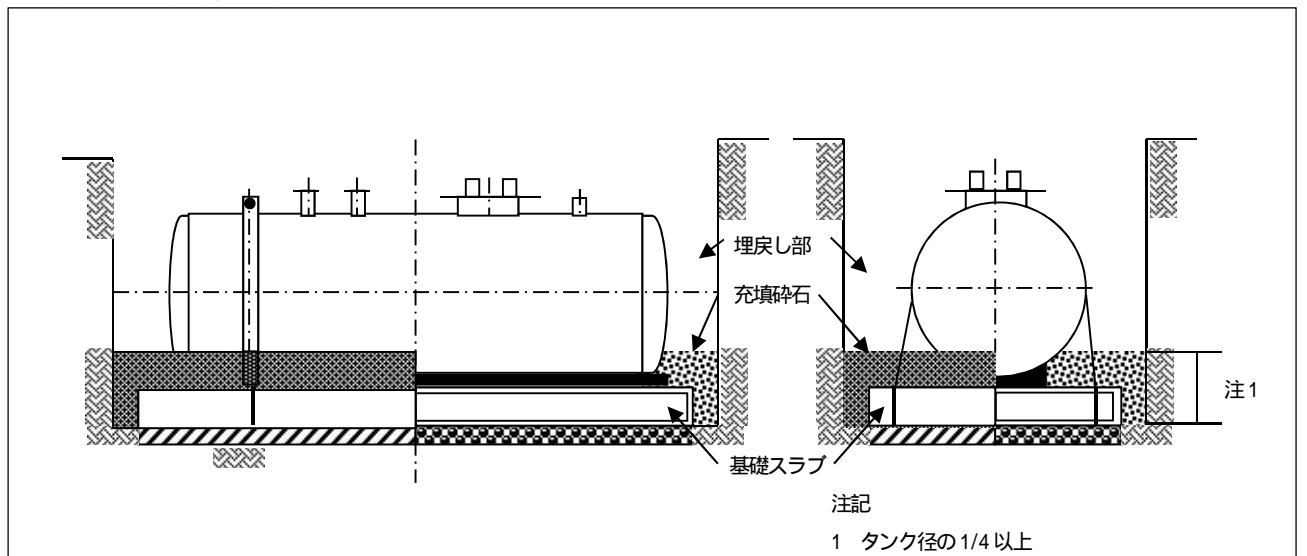
<図 3 - 2 充填碎石施工図>
