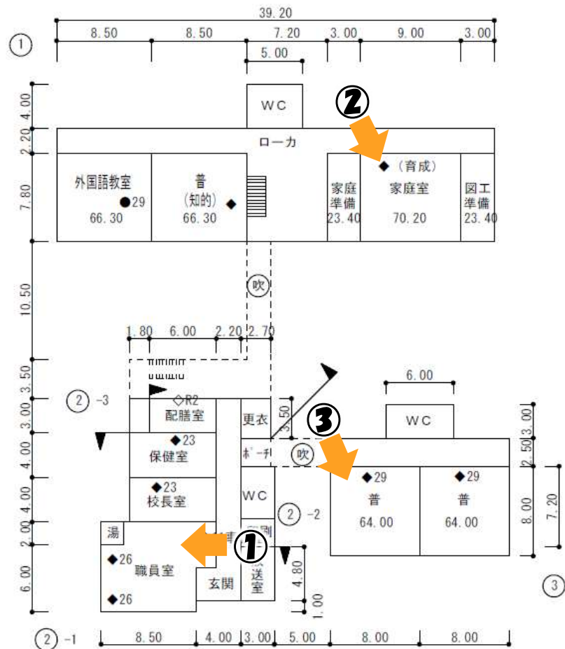
【1階 平面図】
