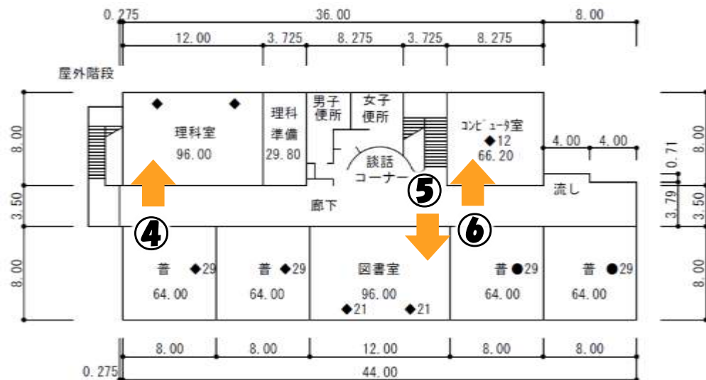
【2階 平面図】
