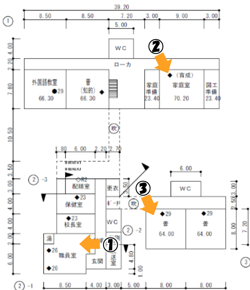
【1階 平面図】
