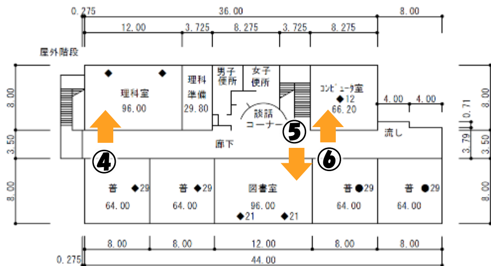
【2階 平面図】
