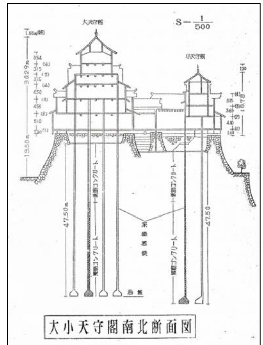
天守閣断面図 (昭和35年資料より)
