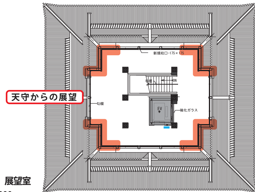
5階 平成 S=1/200
