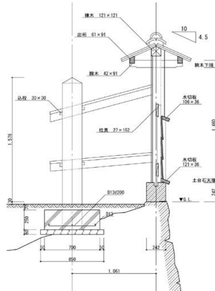
図4 続塀の控柱据付図
