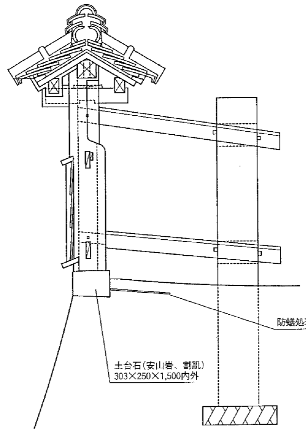
図3 奉行丸塀の控柱据付図 （『特別史跡熊本城跡西出丸一帯復元工事報告書』、熊本市、2005年）
