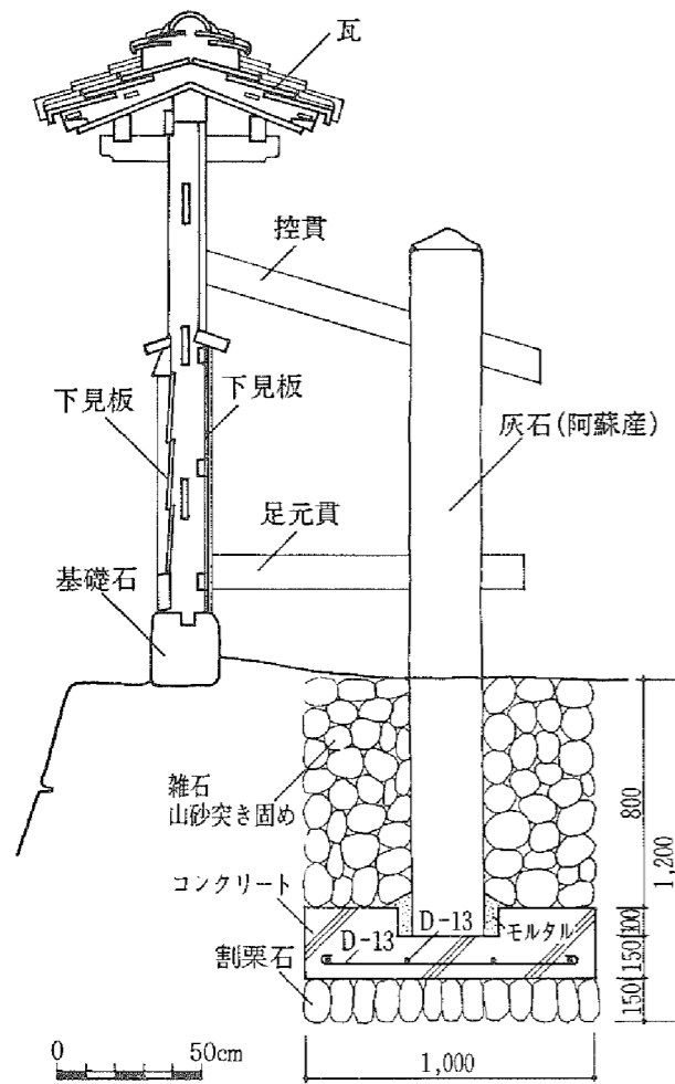
図1 長塀の控柱据付図 （『重要文化財熊本城監物櫓・長塀修理工事報告書』、熊本市、1979年）
