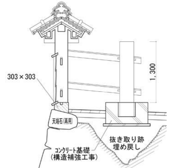
図7 平左衛門丸塀の控柱据付図
