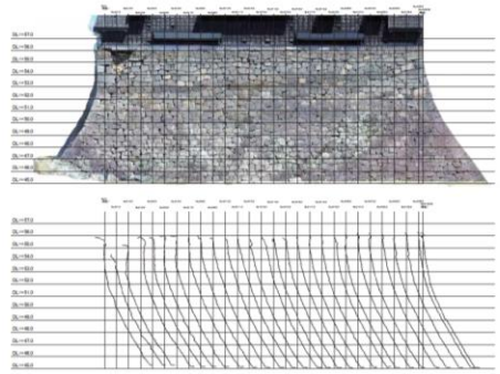
被災後断面図
