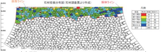
石材問題点分布図・石材控長分布図
