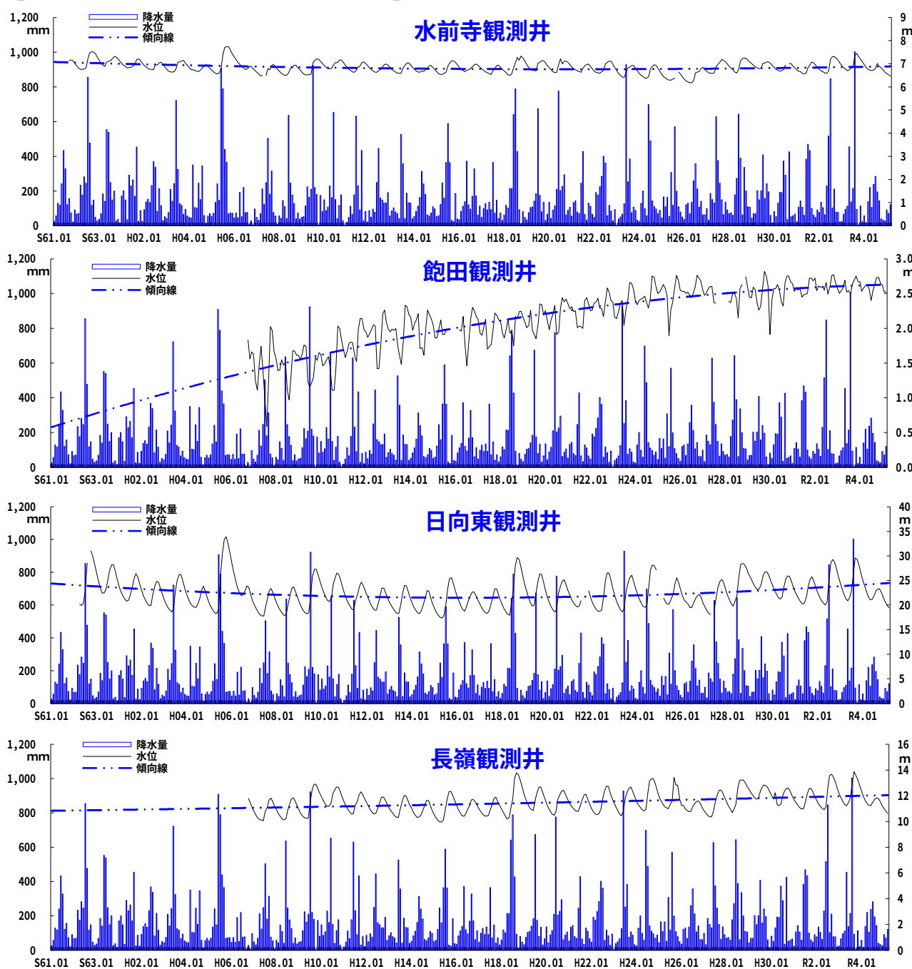
【月別降雨量と観測井の水位経年変化】
