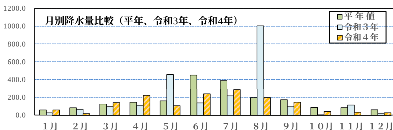
降水量（mm）
