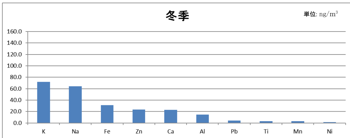
図 1-3-8 各季節の無機成分<成分量の多い 10 種類>(令和 5 年度(2023 年度))
