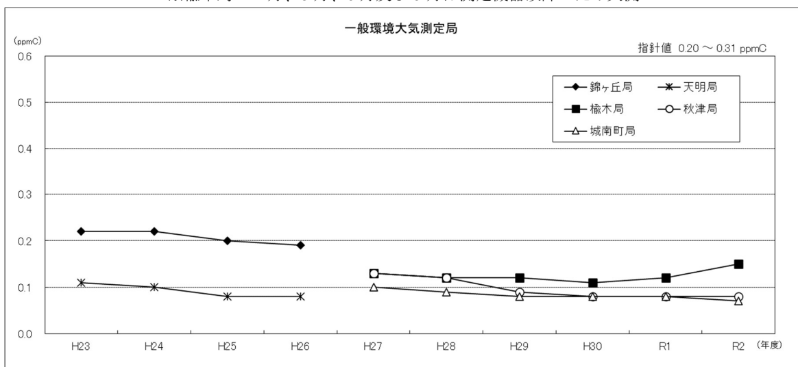
図 1-1-30 非メタン炭化水素の 3 時間値 (6~9 時) 年平均値推移 ※参考値として平成 26 年度(2014 年度)まで測定を行っていた錦ヶ丘及び天明局の年平均値を記載。
