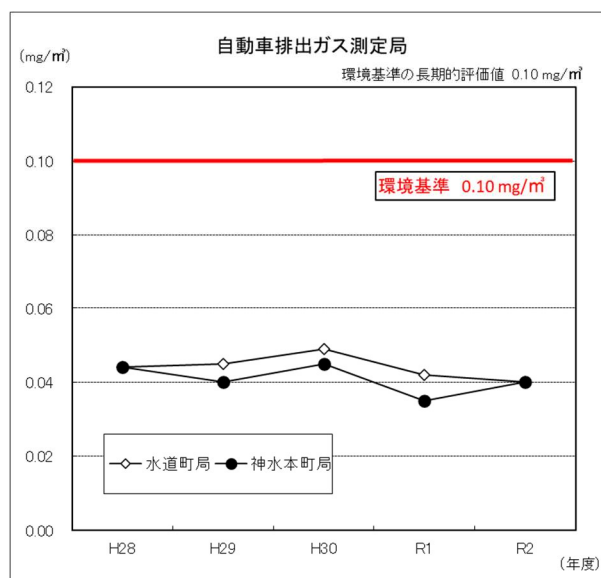
図 1-1-14 浮遊粒子状物質日平均値の2%除外値の推移
