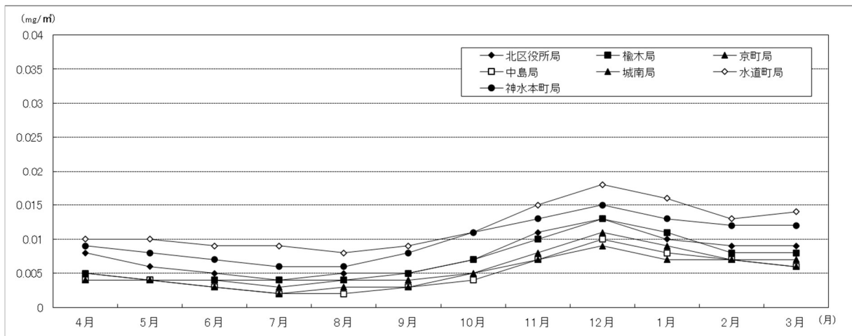
図 1-1-8 二酸化窒素の日平均値推移(令和2年度(2020年度))の月別
