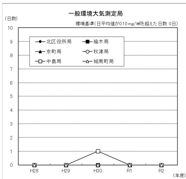
図 1-1-12 浮遊粒子状物質の短期評価(日平均値が 0.10 mg/m 3 を超えた日数)の推移
