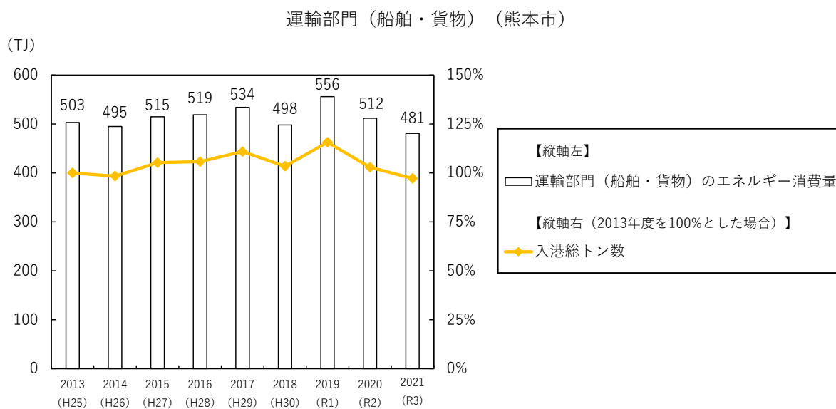
図 20 運輸部門（船舶・貨物）のエネルギー消費量の推移
