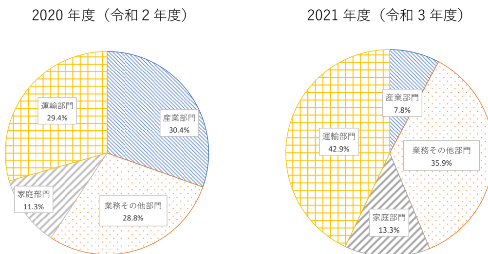
図 6 部門別 CO 2 排出量の構成比（2021 年度（令和 3 年度）との比較）
