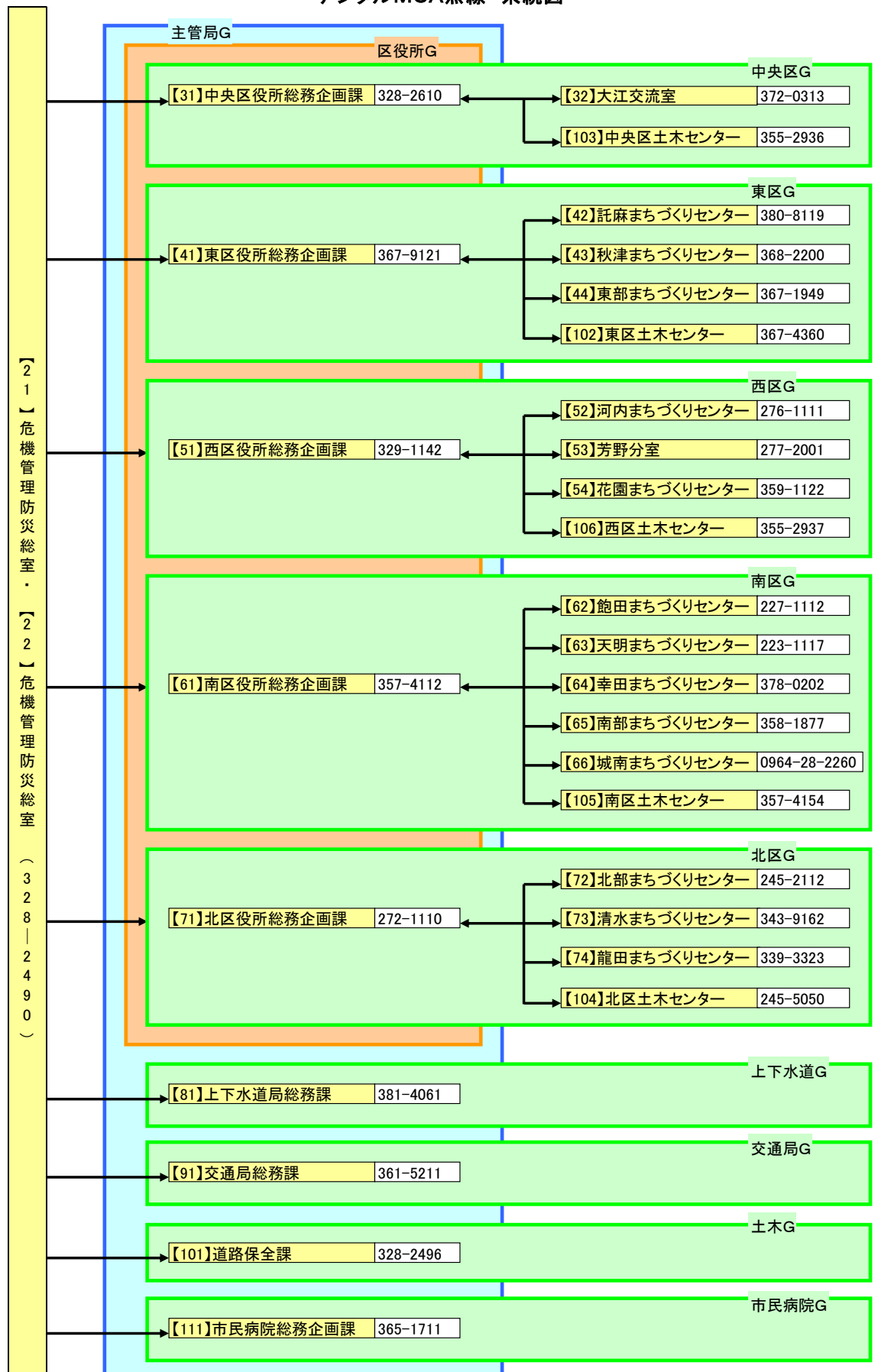
デジタルMCA無線 系統図
