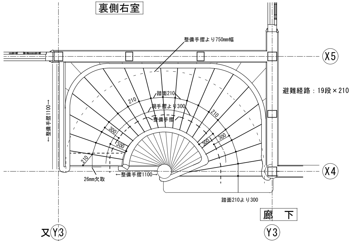
階段踏面検討図
