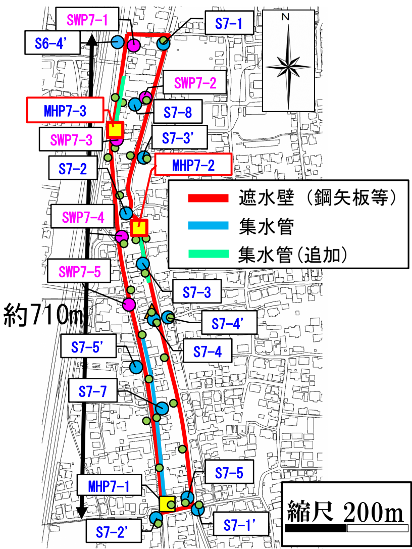
観測位置平面図
