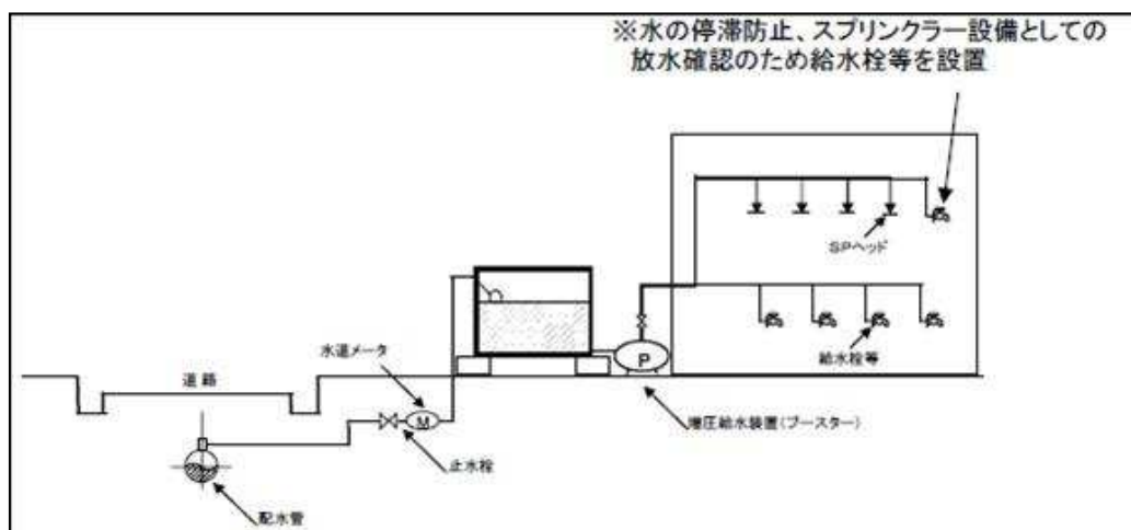
《直結・受水槽補助水槽併用式の例》
