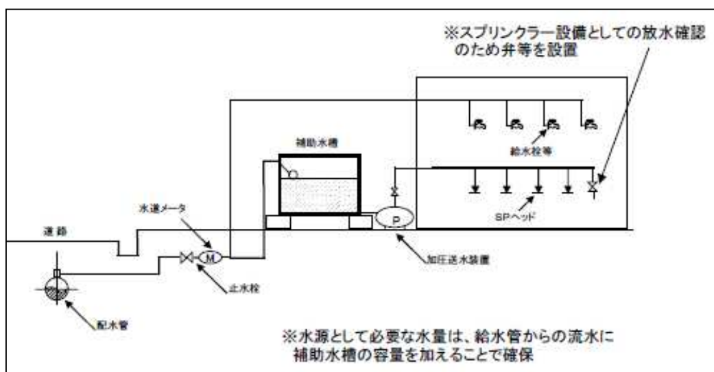
《直結・受水槽補助水槽併用式の例》
