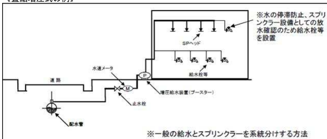
《直結増圧式の例》
