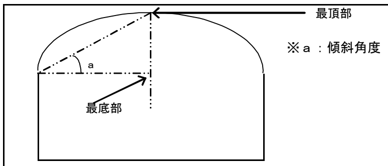
《円形天井の傾斜角度の例》
