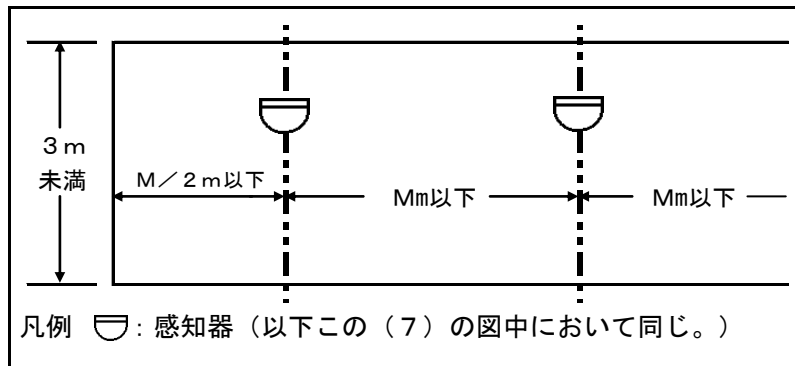
《細長い居室等に感知器を設ける場合の例》
