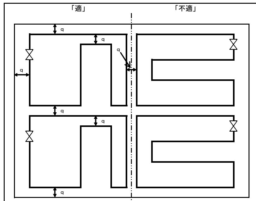
《傾斜天井頂部の空気管の設置例》
