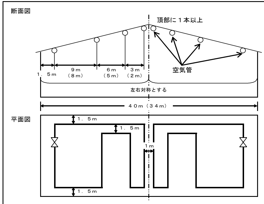
《傾斜天井頂部の空気管の設置例》
