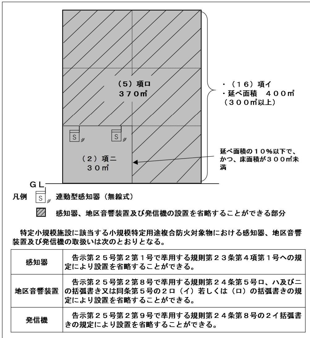
小規模特定用途複合防火対象物に設ける特定小規模施設用自動火災報知設備の構成例
