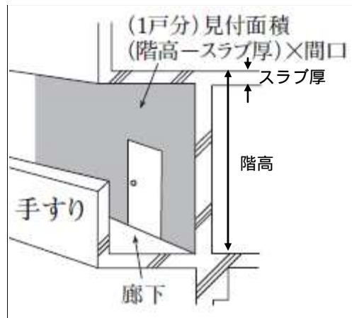
《見付面積の例》
