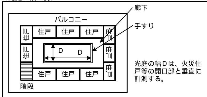
《光庭の幅の例》
