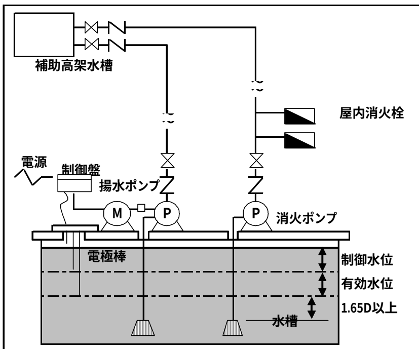
《電極棒による制御方式の設置例》
