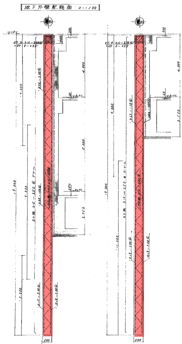
图 3-4 地中連続壁配筋図（立断面図）
