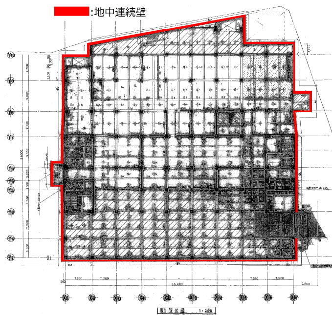
图 3-3 B1 階伏図
