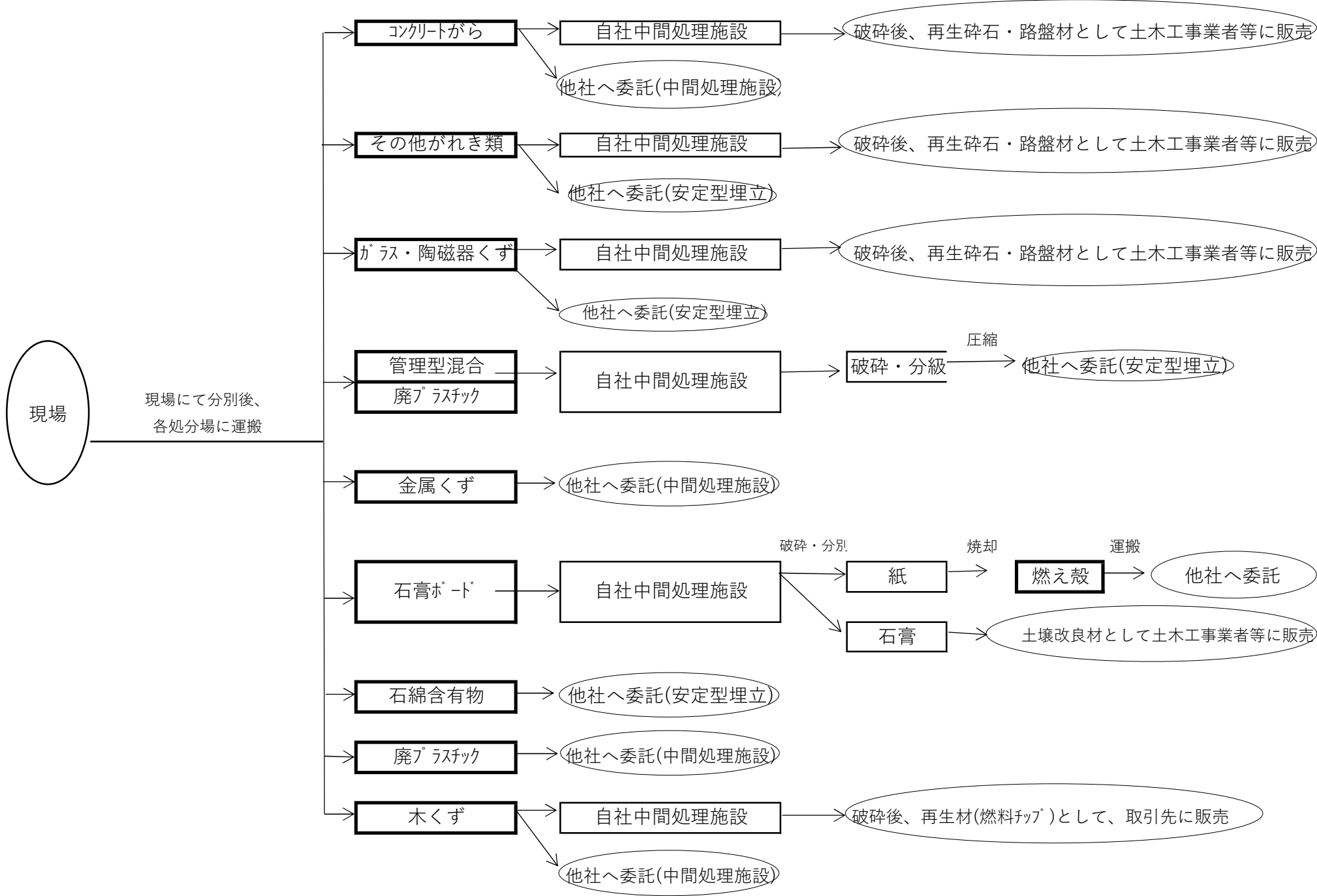
※別紙・産業廃棄物の一連の処理の工程
