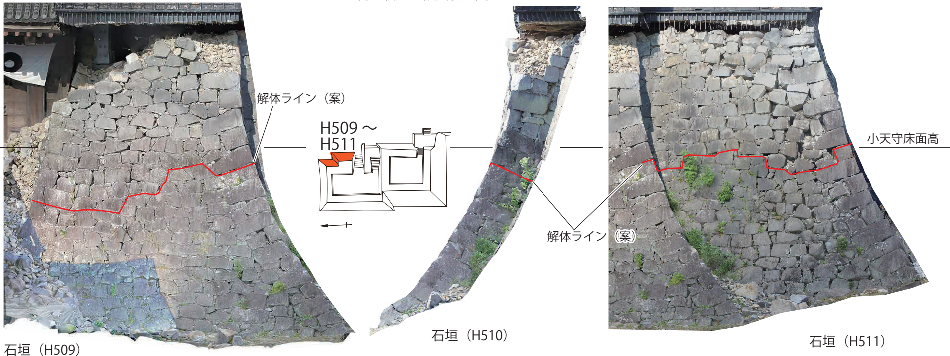
石垣解体範囲案図
