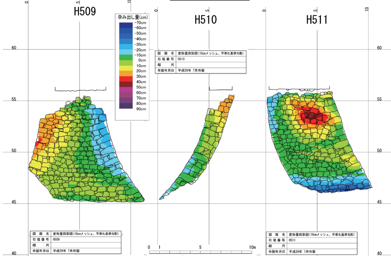
変形量段彩図 (10cm メッシュ、平準化基準勾配)
