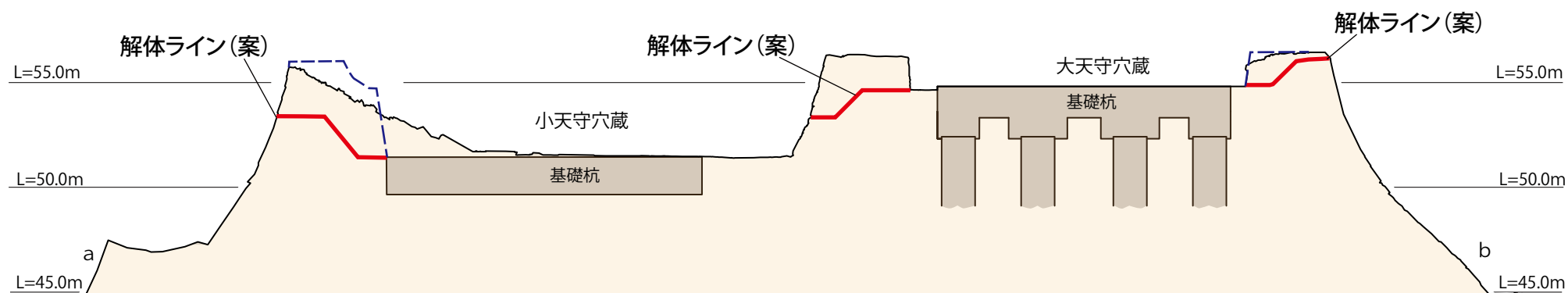
天守南北方向の断面
