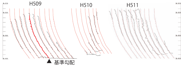
垂直断面図
