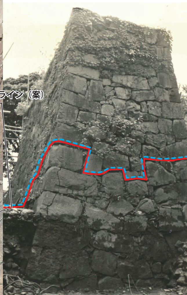
小天守入口南面石垣（H500）・同穴蔵東面石垣（H501）
