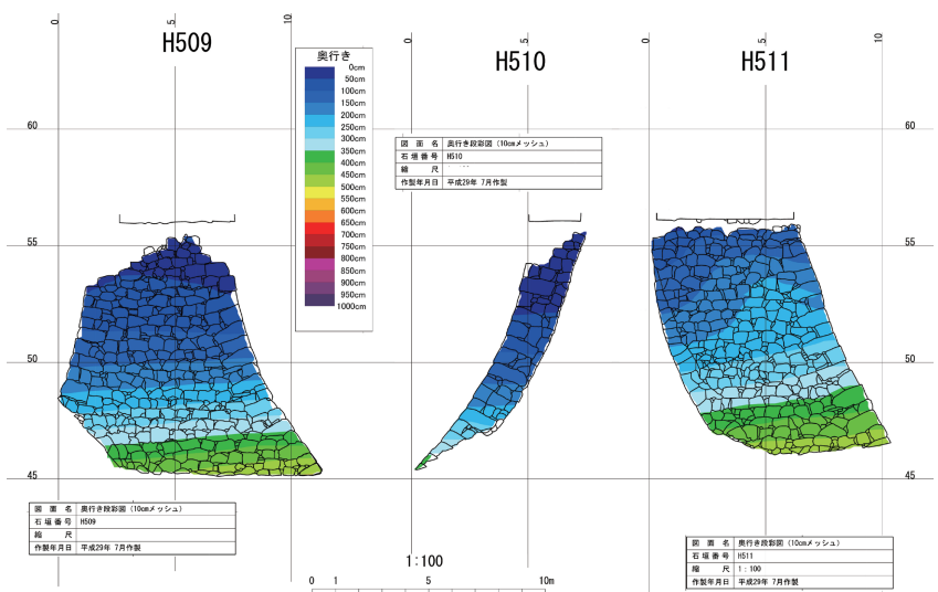
奥行き段彩図 (5mm 点群)
