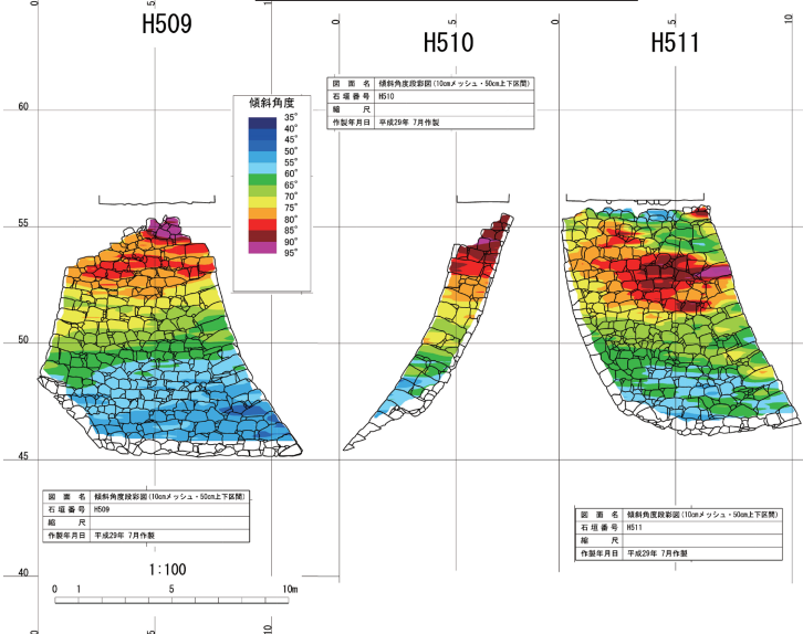
傾斜角度段彩図 (10cm メッシュ・50cm 上下区間)
