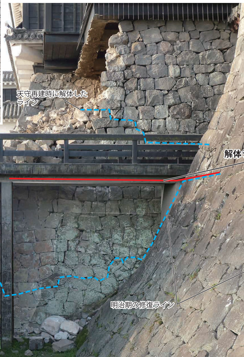
小天守入口南面石垣（H500）
