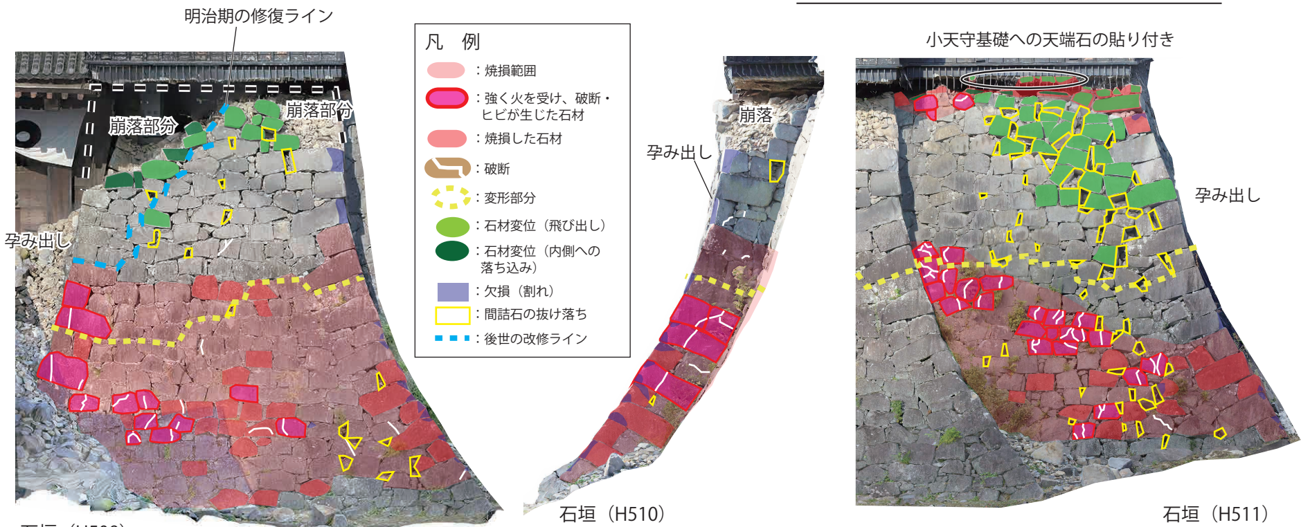
石垣履歴・被災状況図
