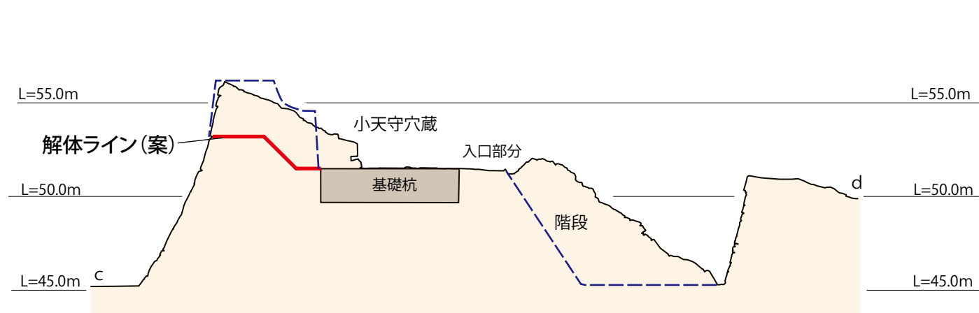
小天守東西方向の断面
