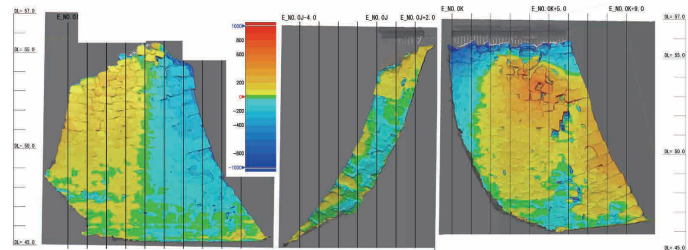
変形量段彩図 (5mm 点群、1 断面基準勾配)
