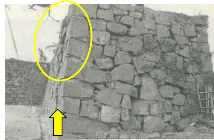
石垣上の樹木による変状（奉行所）
