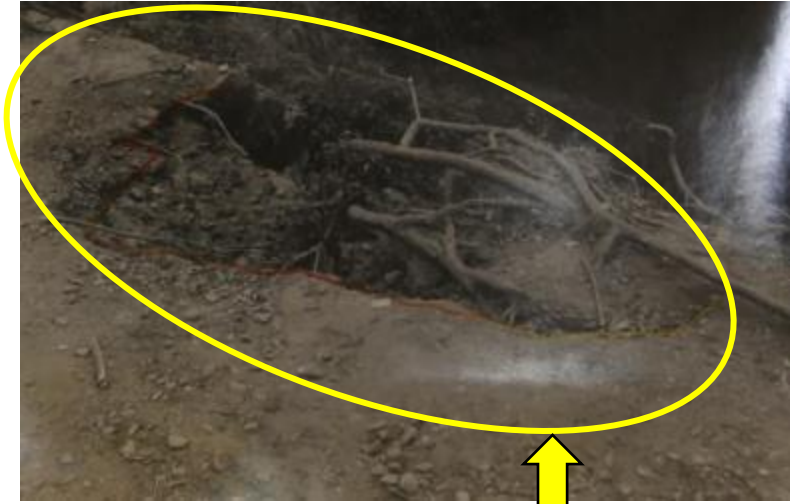
倒木により加藤神社石垣天端石が崩落
