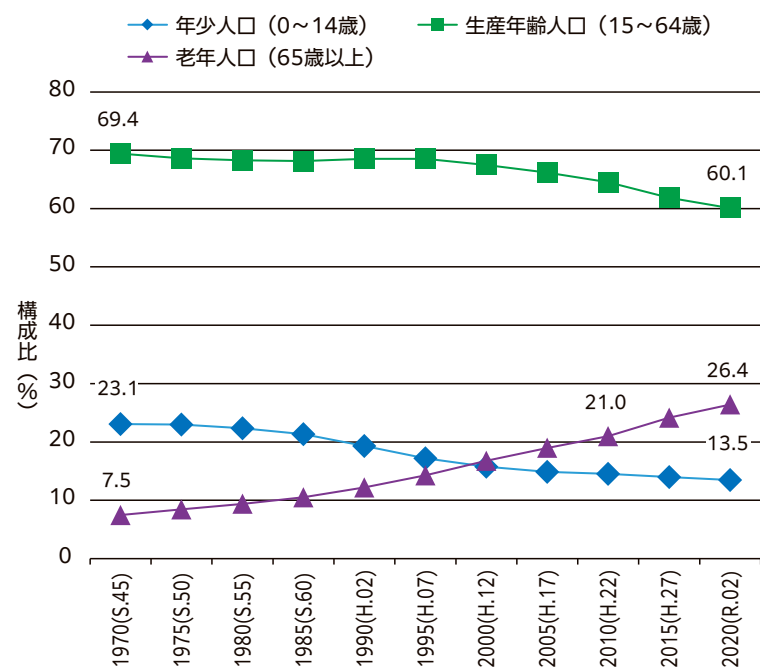
年齢3区分別人口構成比(合併組替人口)
