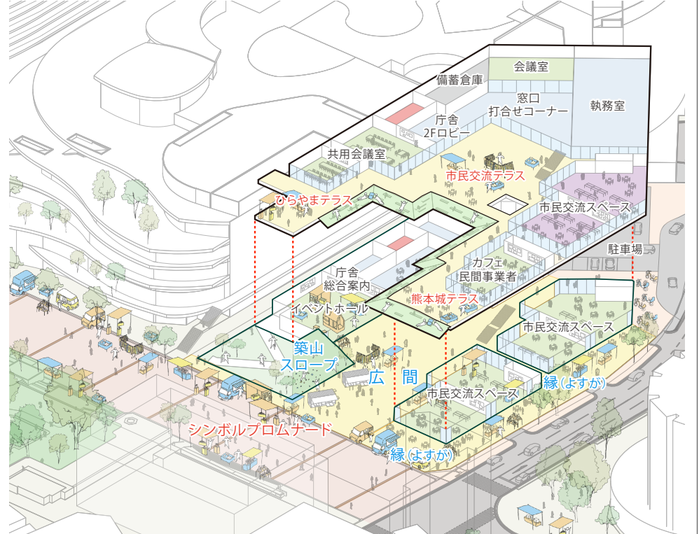
図4-3:様々な市民の居場所をつくる『むすびの間』イメージ
