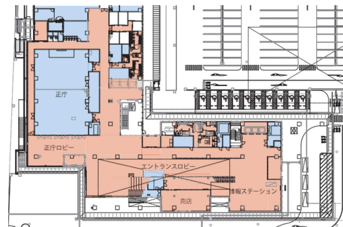
低層棟1階平面図
