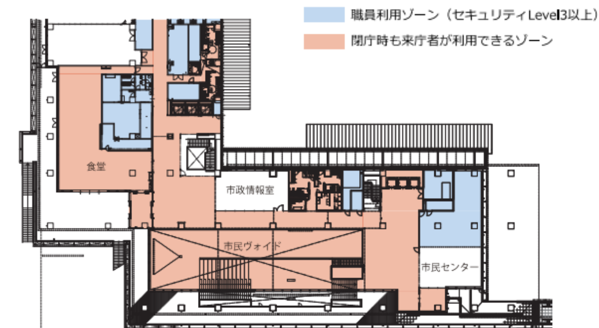
低層棟2階平面図
