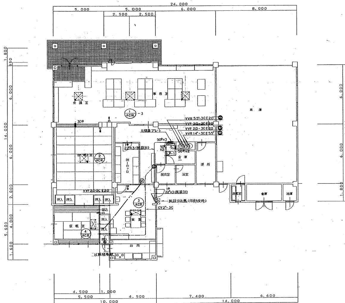
1 階平面図 1/100
