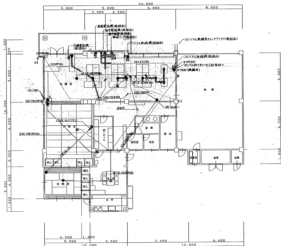
1 階 平 面 図 1/100
