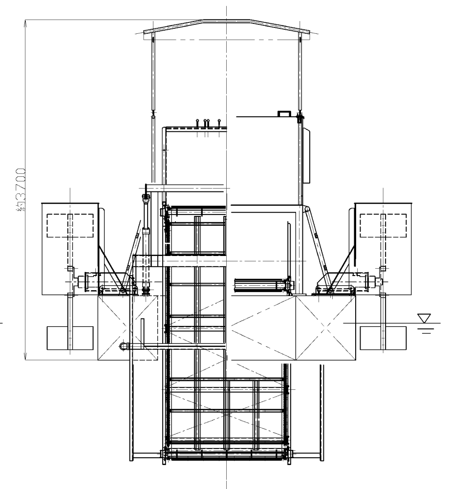
水草回収船 一般配置図（参考）
