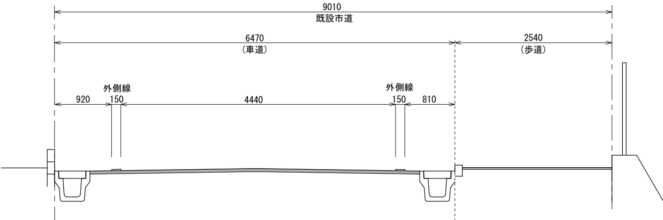
B-B'断面図 S=1:60 既設道路
