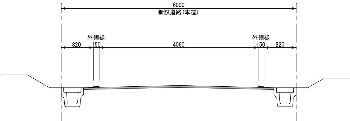
D-D'断面図 S=1:60 新設道路
