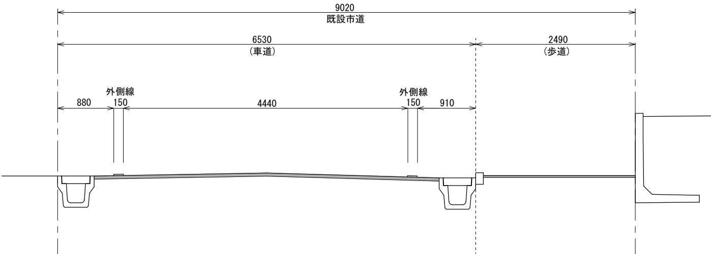
A-A'断面図 S=1:60 既設道路
