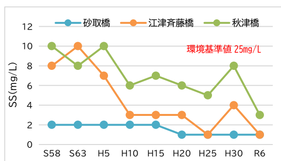
図 3-5 江津湖の SS の推移
