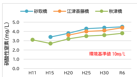
図 3-6 江津湖の硝酸性窒素濃度の推移
