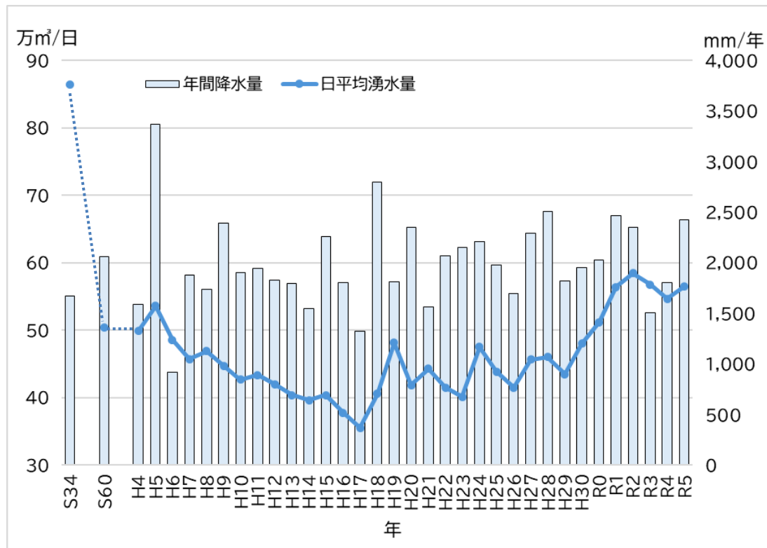
図 3-1 江津湖日平均湧水量の推移
