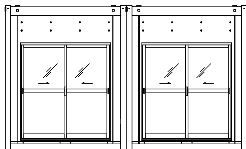
立面図
